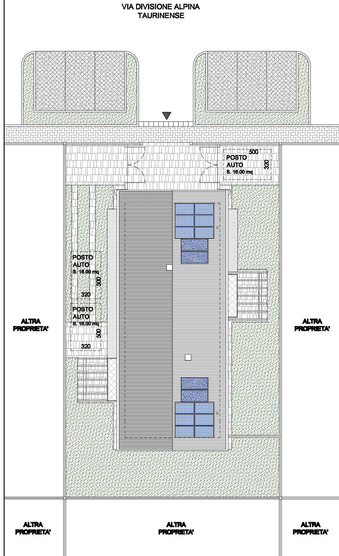
PLANIMETRIA QUOTATA Scala 1:200
